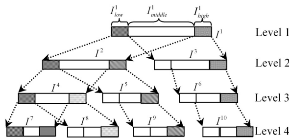
그림 2: 계층적 공간 분할 트리
