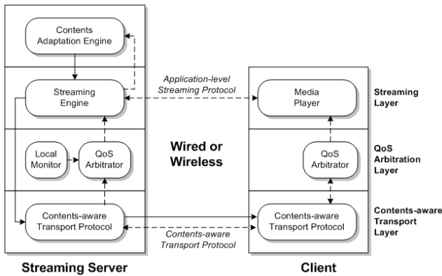
그림 1. 시스템 구조
