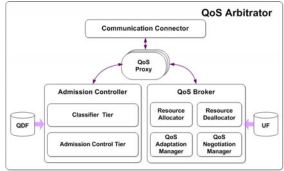
그림 2. QoS Arbitrator
