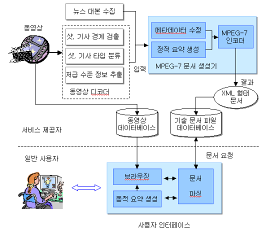
그림 12 시스템 구조
