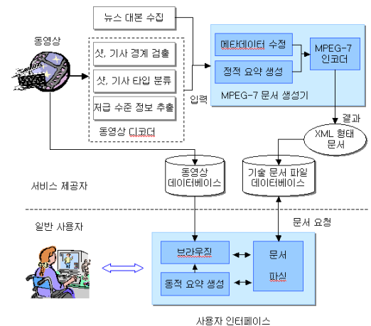
그림 12 시스템 구조
